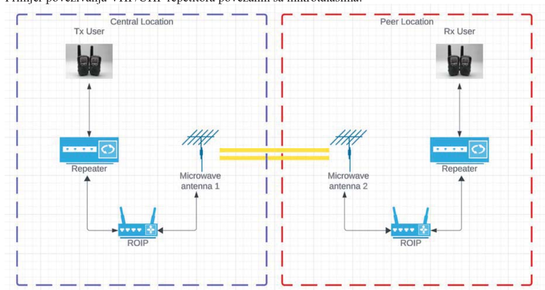
Slika br.1:Povezivanje VHF/UHF repetitora sa mikrotalasima 3
