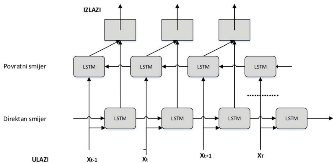
Slika 8. Arhitektura BiLSTM sistema
