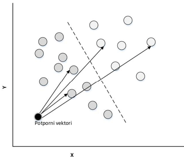
Slika 6. Prostor klasifikacije u SVM metodi
