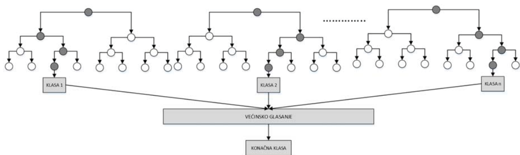
Slika 5. Binarno stablo odlučivanja
