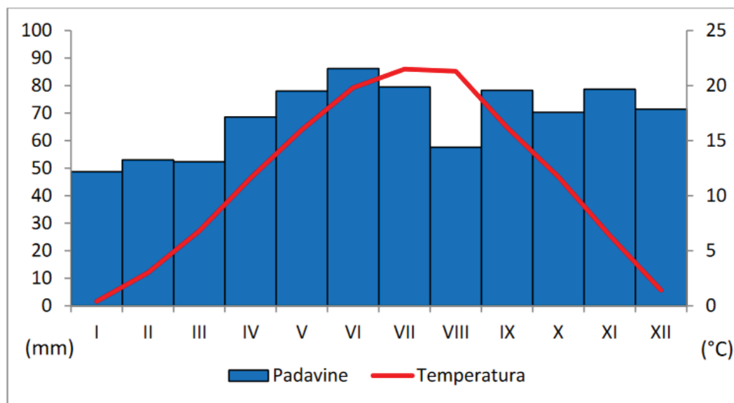
Grafikon br. 1. Prosječne mjesečne vrijednosti temperature vazduha i količine padavina u Zenici od 1991. do 2020. godine
