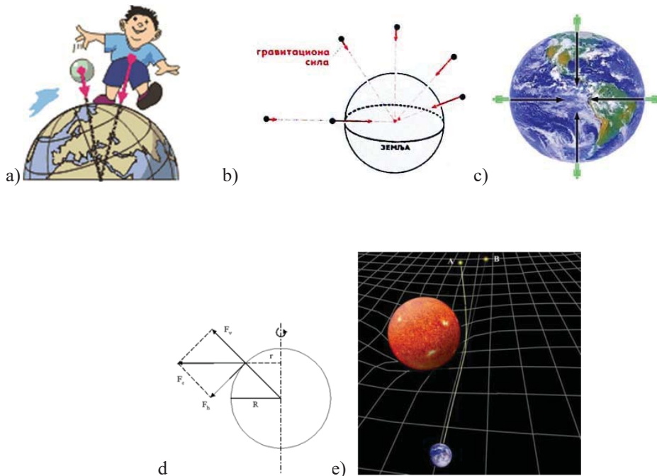
Sl 1. Gravitacija a) Osjećaj težine; b) vektor gravitacione sile; c) Vektor težine čovjeka; d) Utjecaj rotacije Zemlje na težinu tijela; Centrifugalna sila F_c i njene komponente (vertikalna i horizontalna); e) Deformacija prostora prisustvom gravitacije
