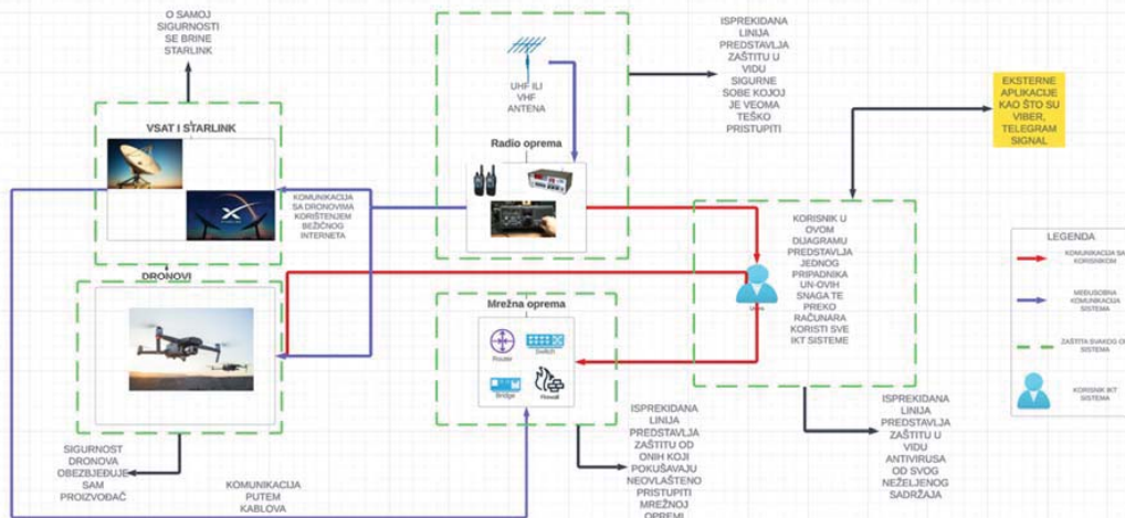
Slika br. 3: Međusobna povezanost IKT sistema u funkciji povećanja pouzdanosti i sigurnosti 5
