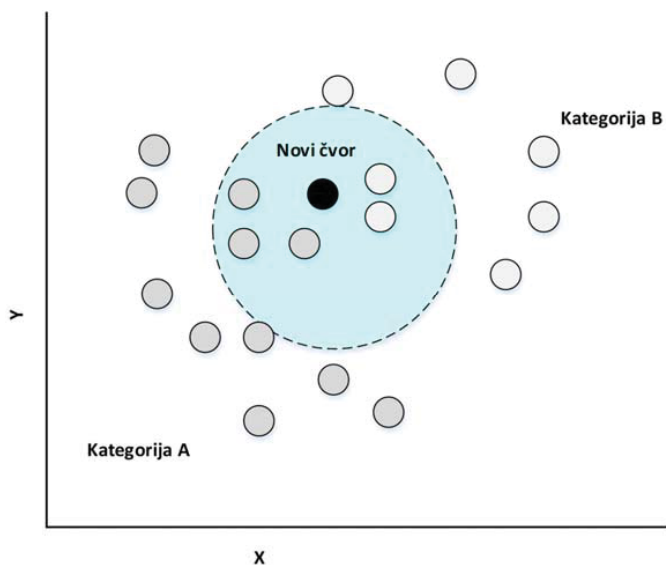
Slika 7. KKN algoritam
