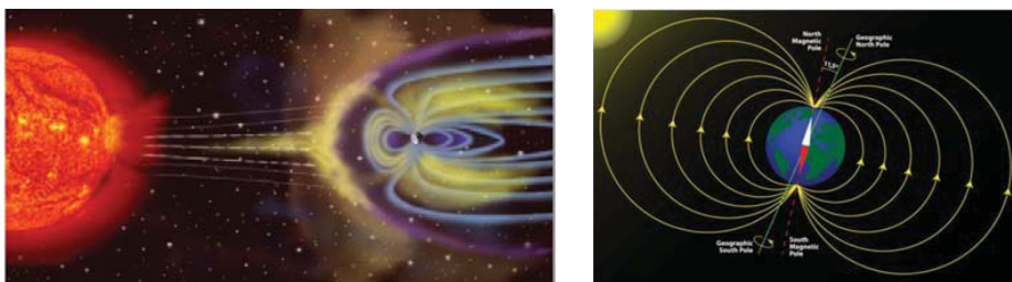
Slika 3. Prikaz magnetnog polja zemlje
